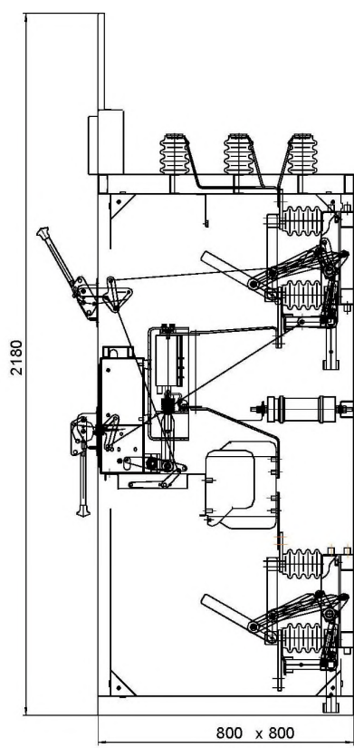
Общий вид и габаритные размеры КСО «Кедр»
